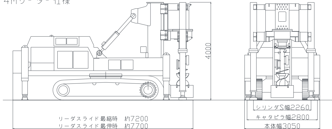
側面図
