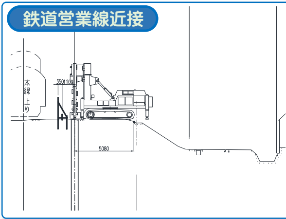
削孔
